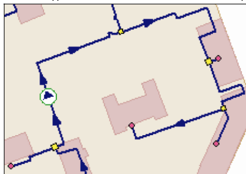
Рисунок 9.7. Тепловая сеть
